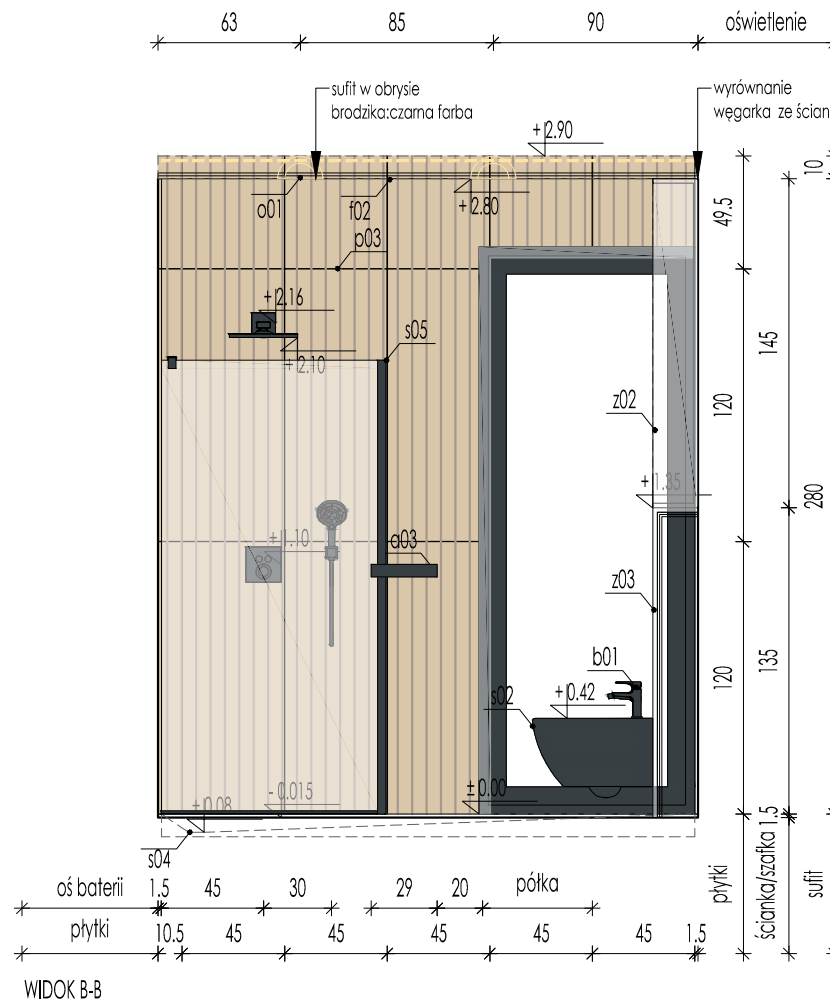
WIDOK B-B
